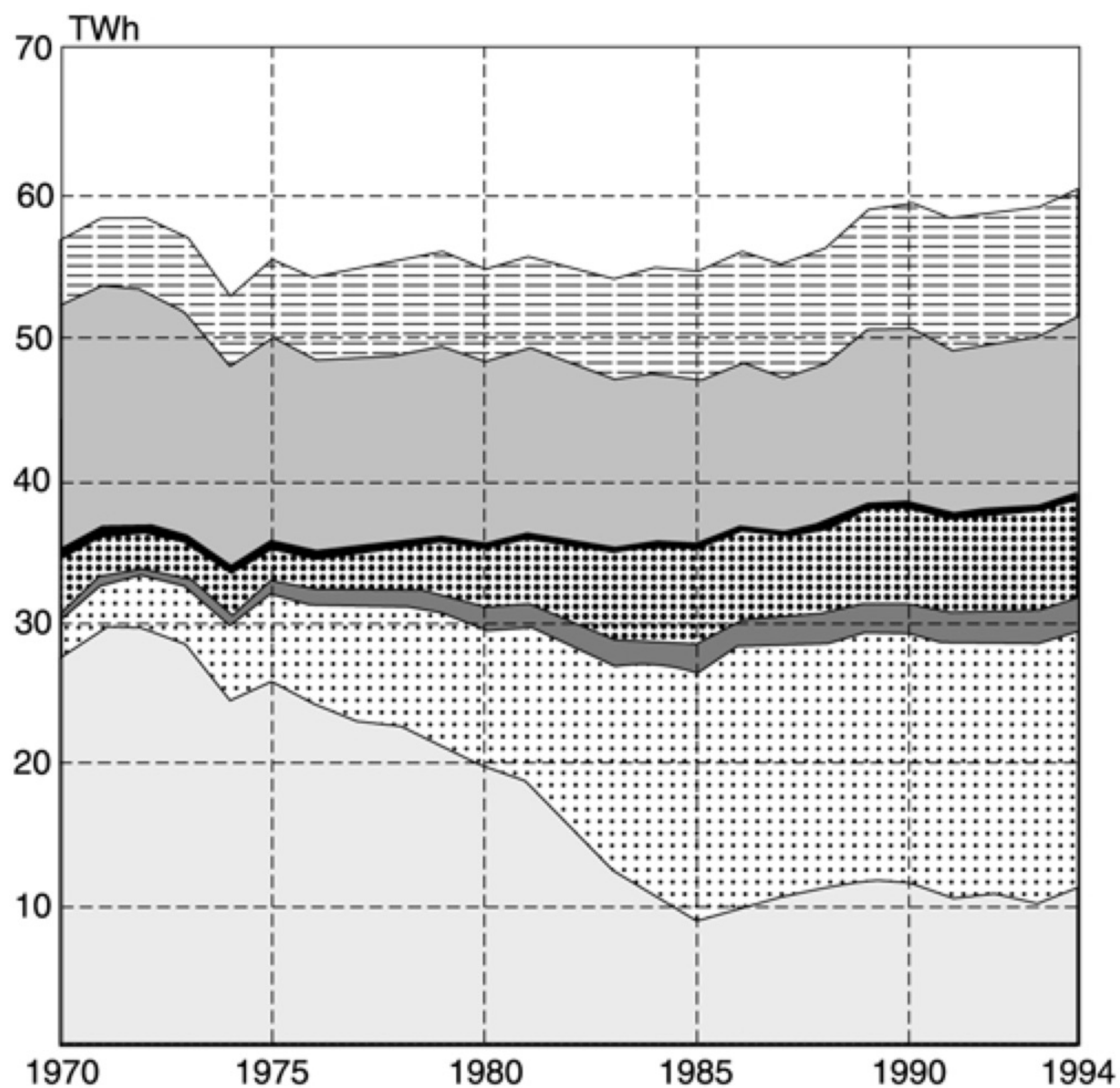
Energianvändningen i småhus uppdelad på energibärare. TWh.
