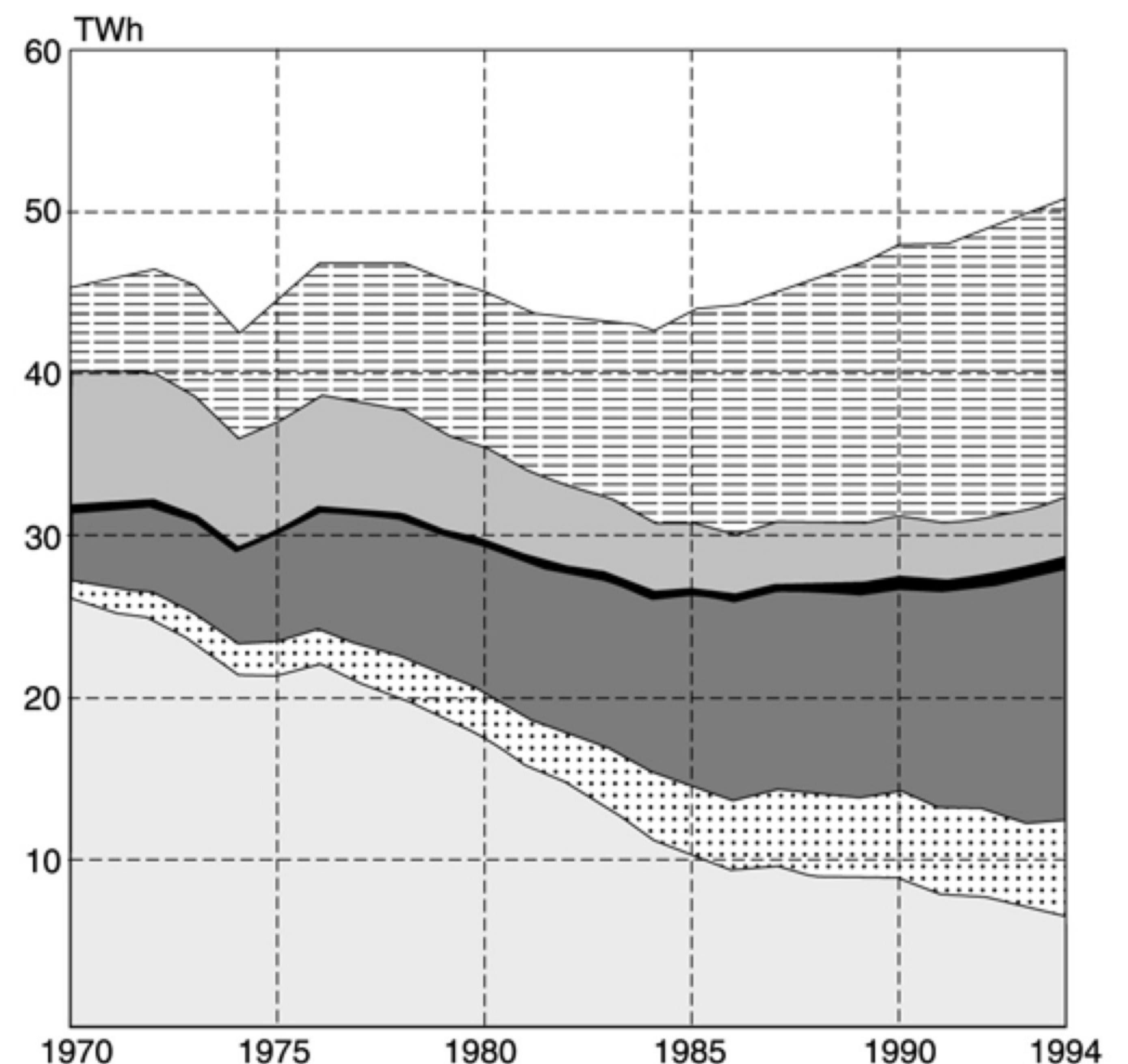
Energianvändningen i servicelokaler uppdelad på energibärare. TWh.
