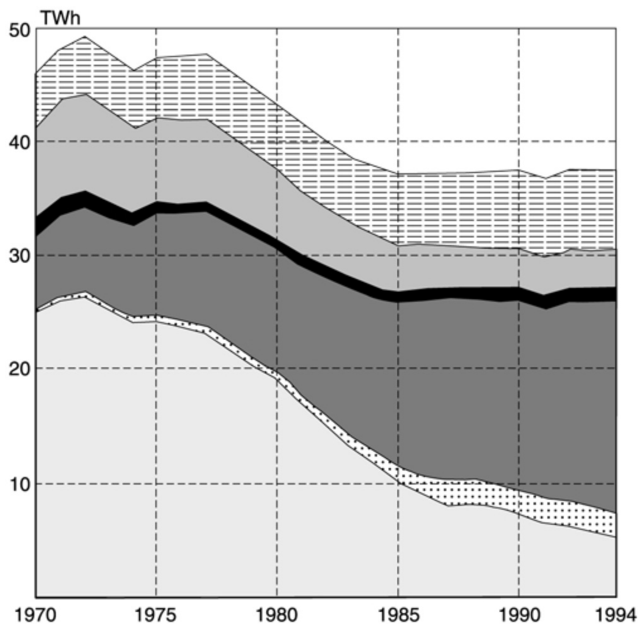
Energianvändningen i flerbostadshus uppdelad på energibärare. TWh.
