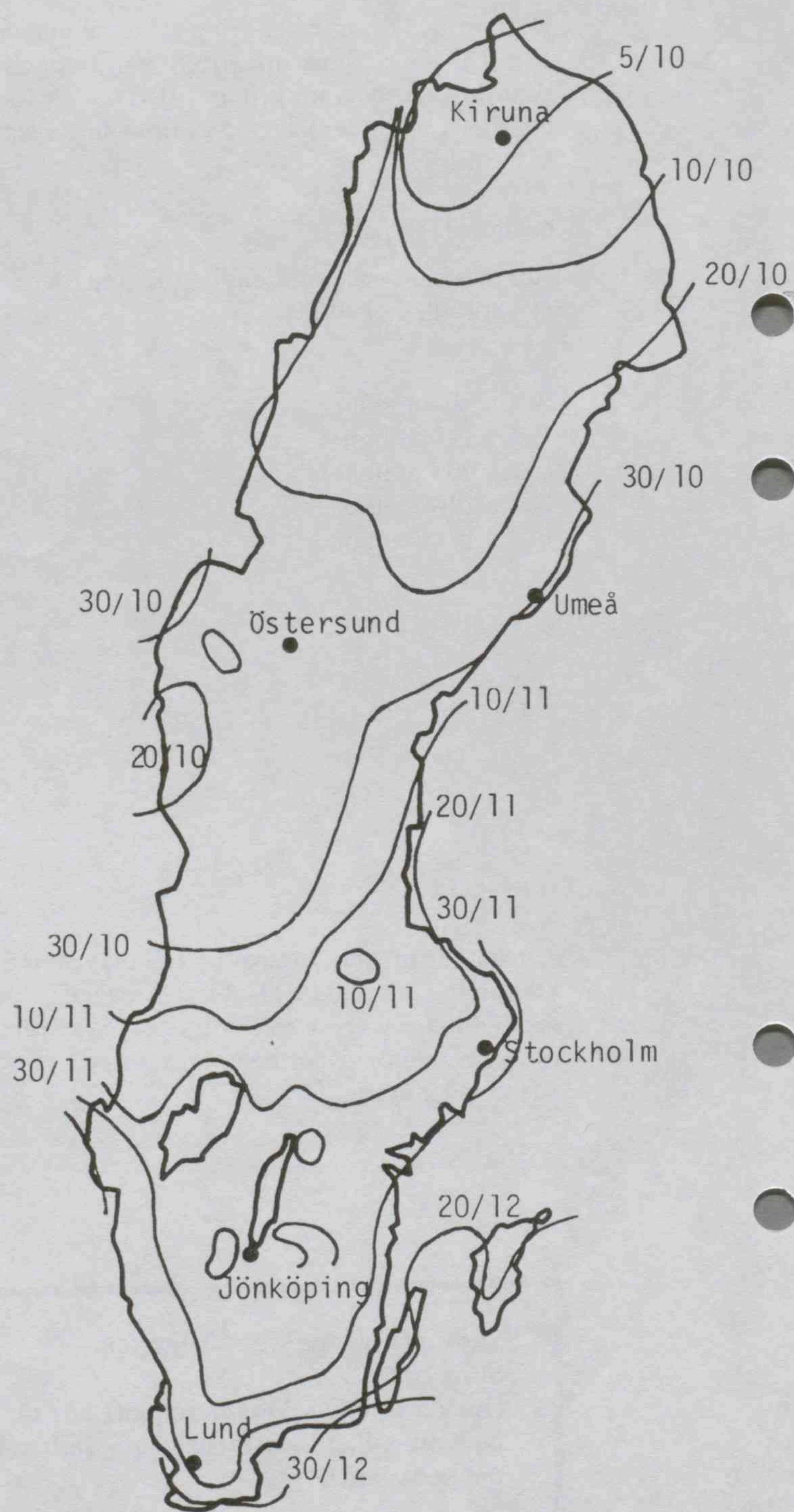
Vinterns ankomst. Medeltemperaturen sjunker till \pm 0^{\circ}\text{C} .
